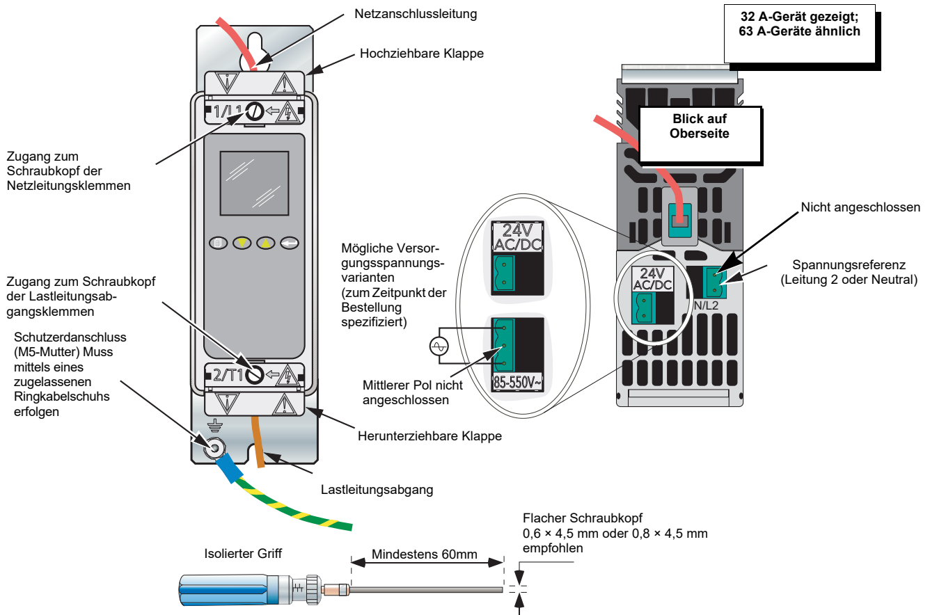
Einzelheiten zum Schraubendreher/Schraubenschlüssel für Leitungs- und Lastabschlüsse
