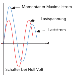
Abbildung 21 Definition bei verzögerter Auslösung
