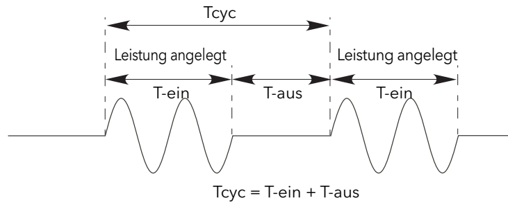
Abbildung 14 Impulsgruppe mit festem Intervall
