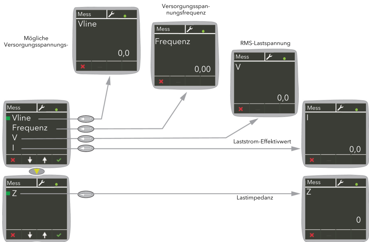
Abbildung 17 Messwert-Menü
