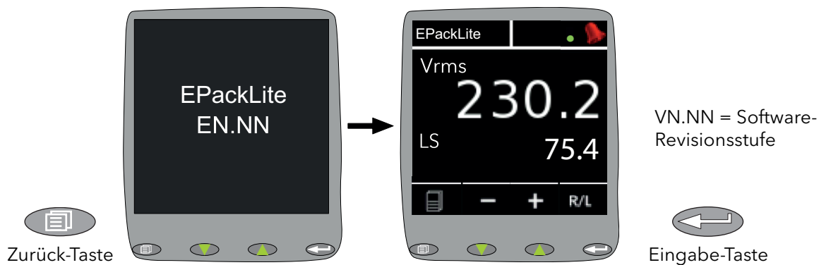
Abbildung 16 Initialisierungsbildschirme
