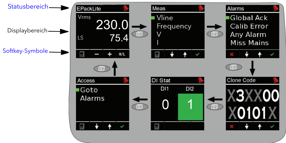
Abbildung 11 Bedienoberfläche
