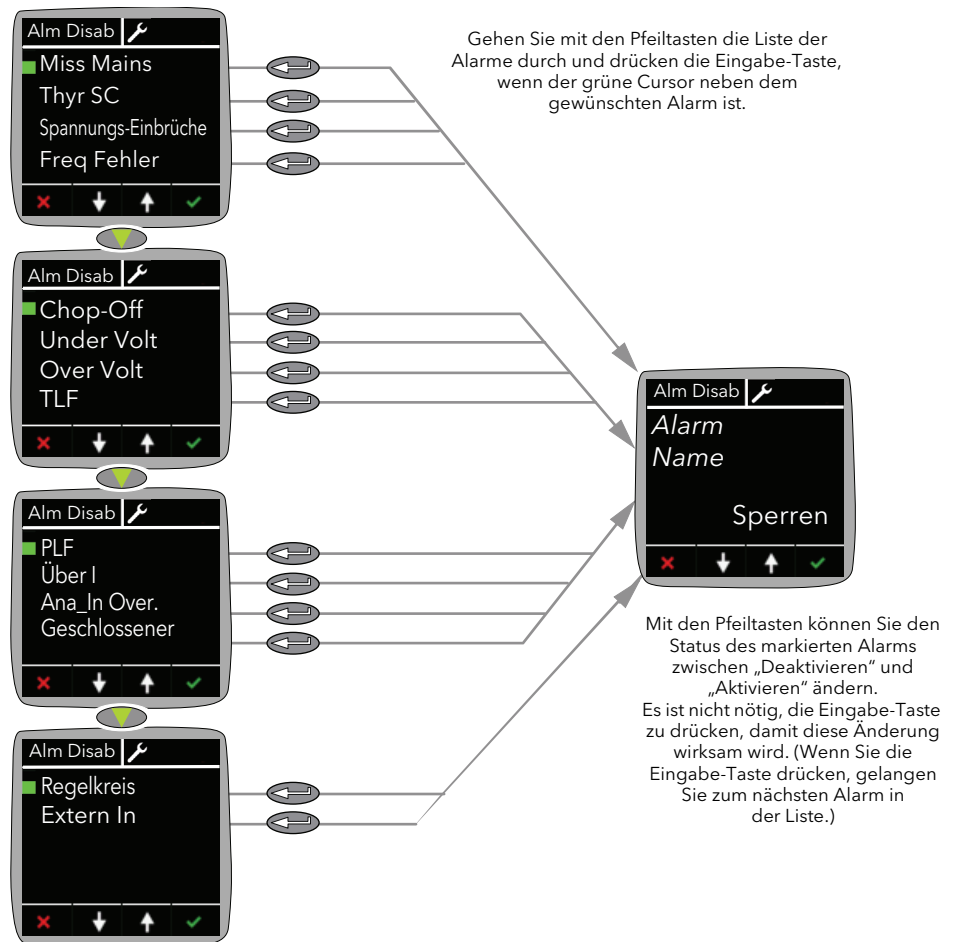
Abbildung 25 Alarmdeaktivierungsmenü
