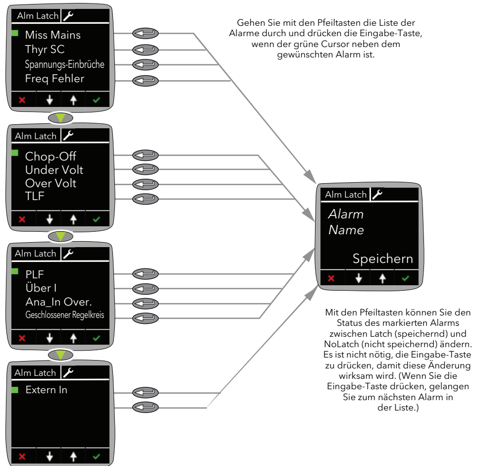
Abbildung 26 Alarmspeichermenü
