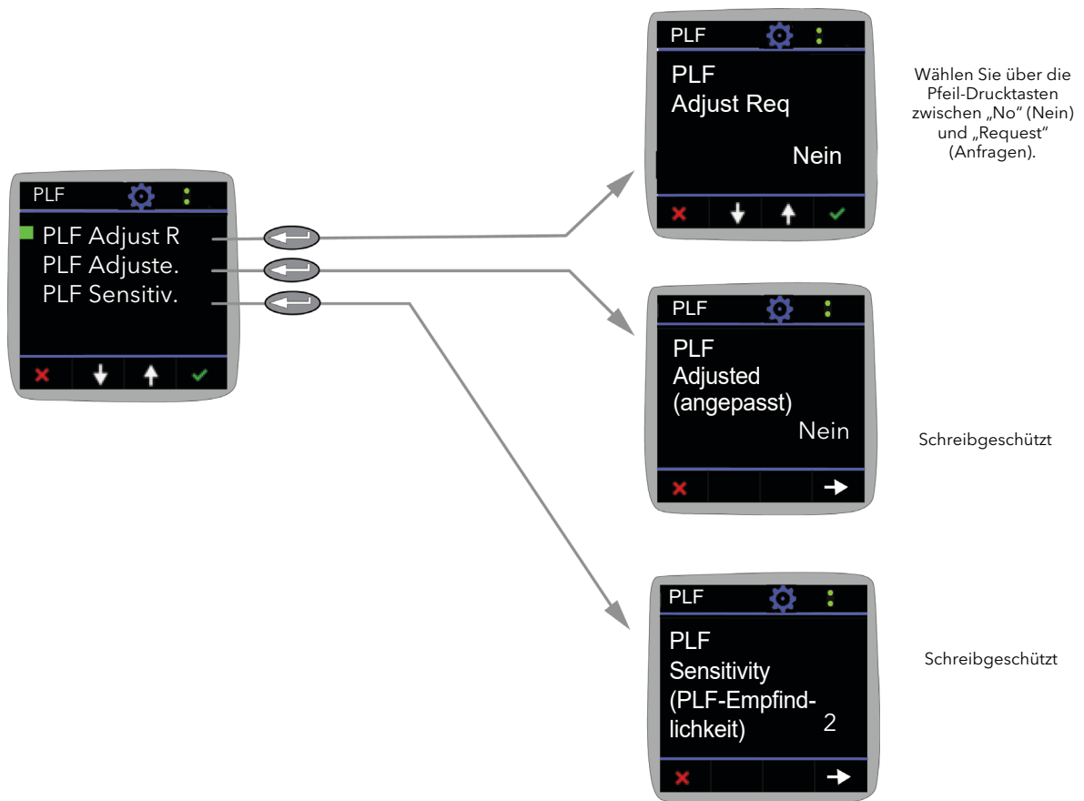
Abbildung 22 PLF-Menü
