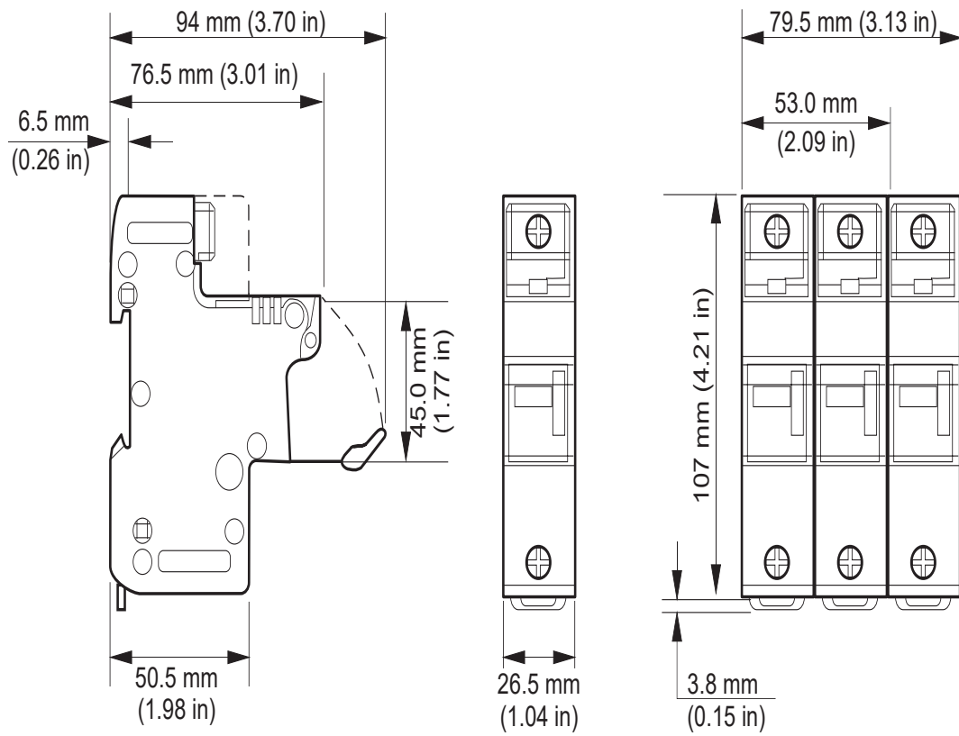
Abbildung 34 Sicherungshalterabmessungen: US141 (14x51 mm)
