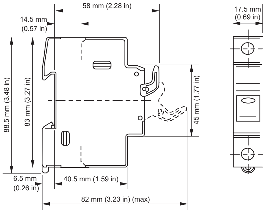
Abbildung 32 Sicherungshalterabmessungen: US101 (10x38 mm)
