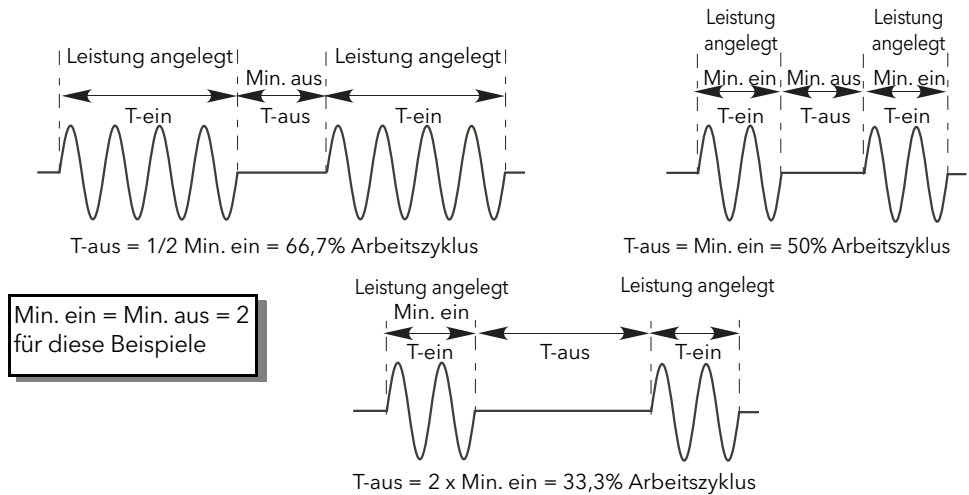
Abbildung 15 Impulsgruppe mit variablem Intervall
