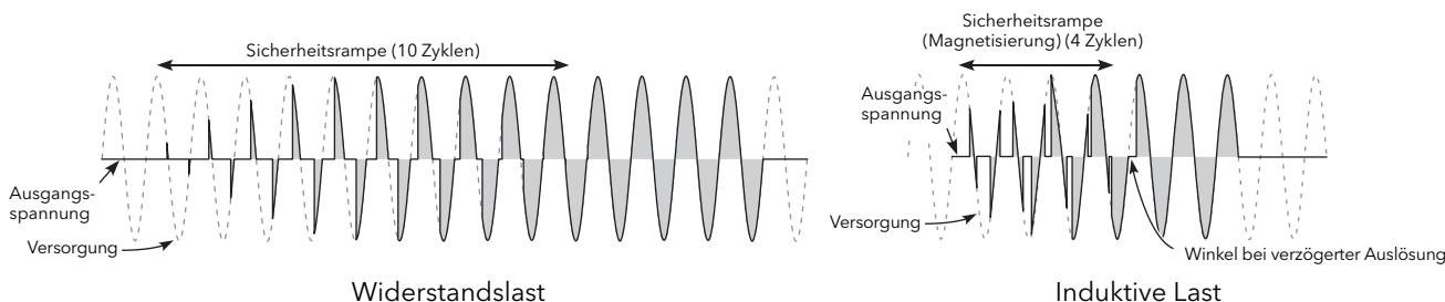
Abbildung 19 Beispiele für Sicherheitsrampen (Impulsgruppenbetrieb)
