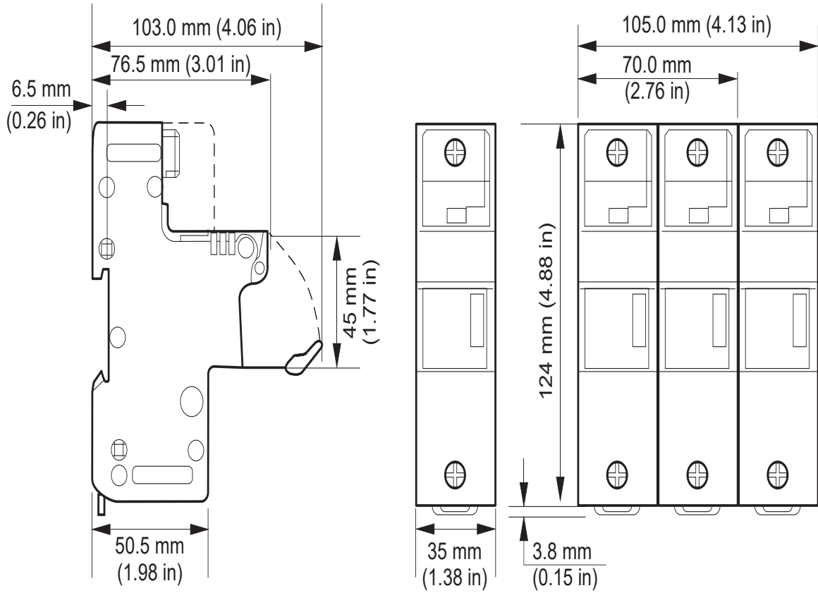
Abbildung 35 Sicherungshalterabmessungen: US221 (22x58 mm) Sicherungshalter-
