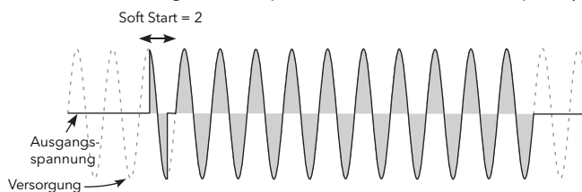
Abbildung 19 Beispiele für Sicherheitsrampen (Impulsgruppenbetrieb)
