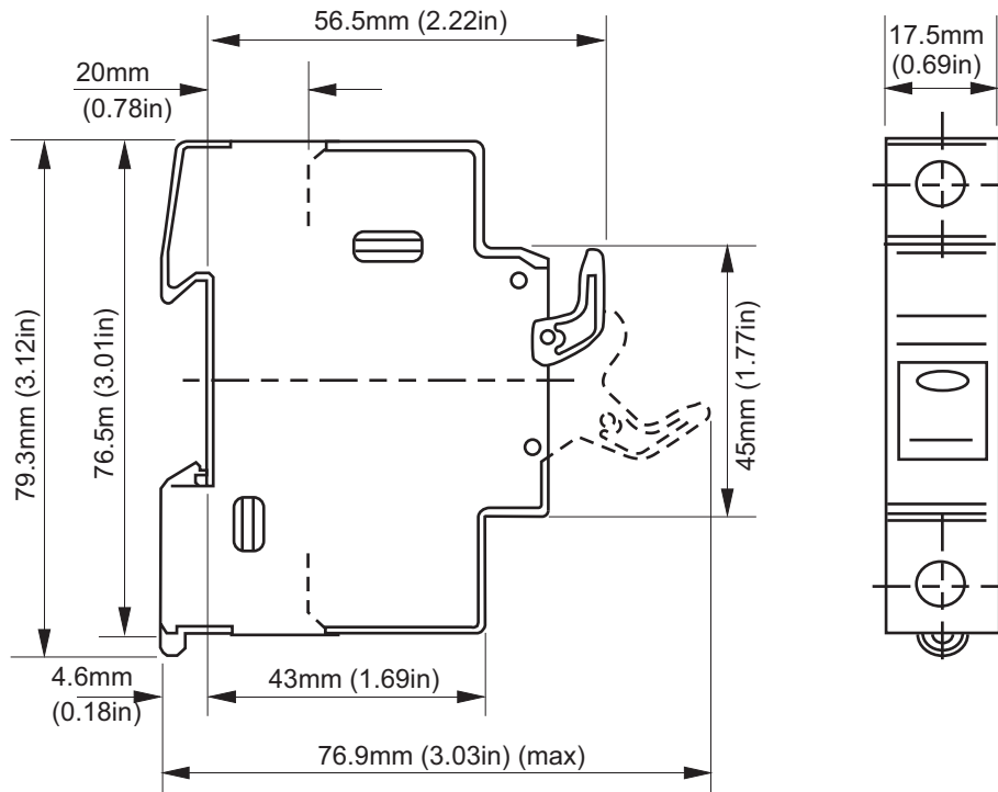
Abbildung 33 Sicherungshalterabmessungen: CUS101 (10x38 mm)
