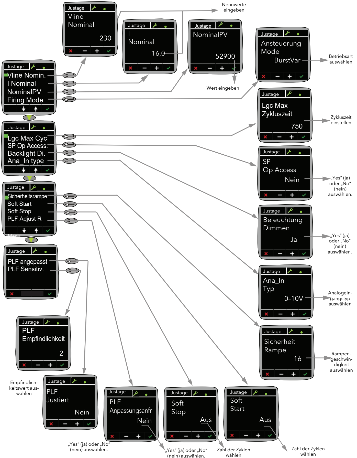
Abbildung 18 Adjust-Menü
