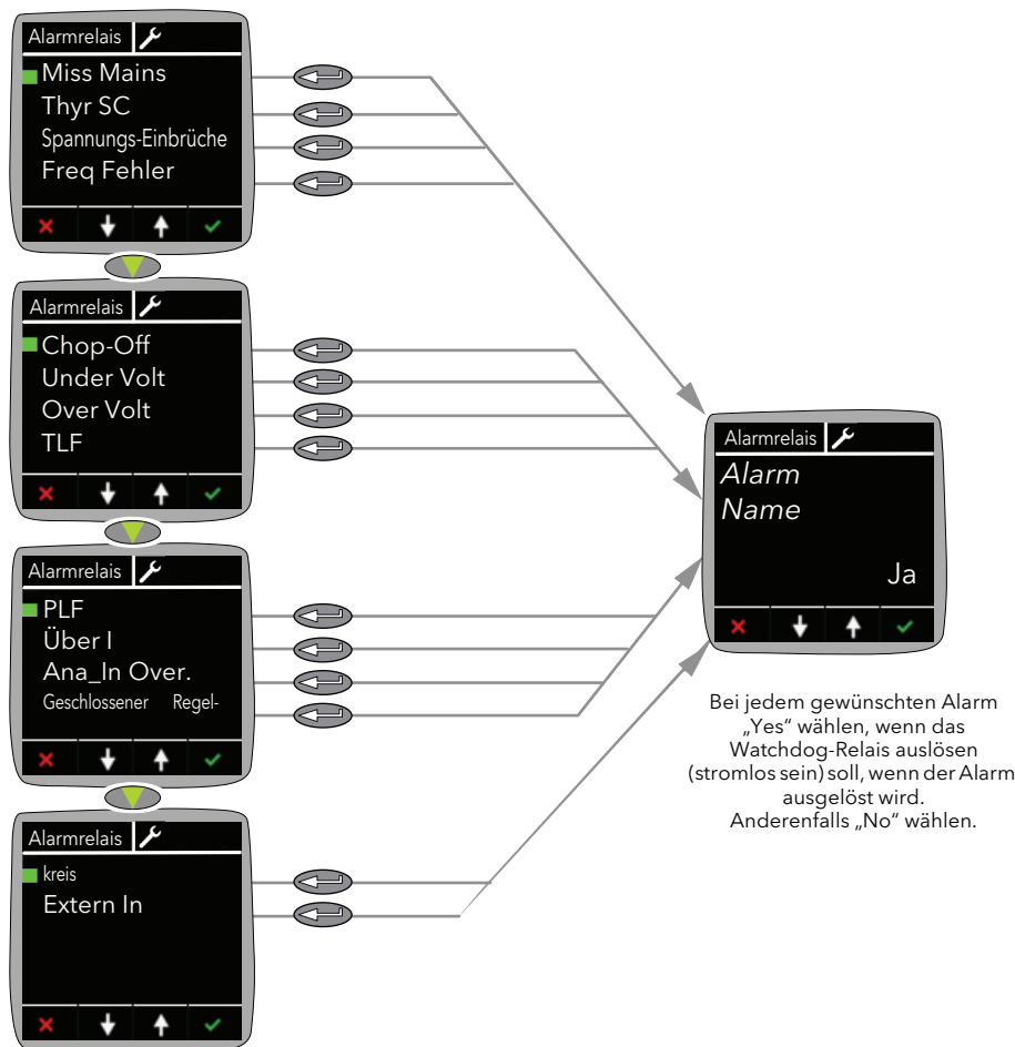
Abbildung 28 Alarmrelaismenü
