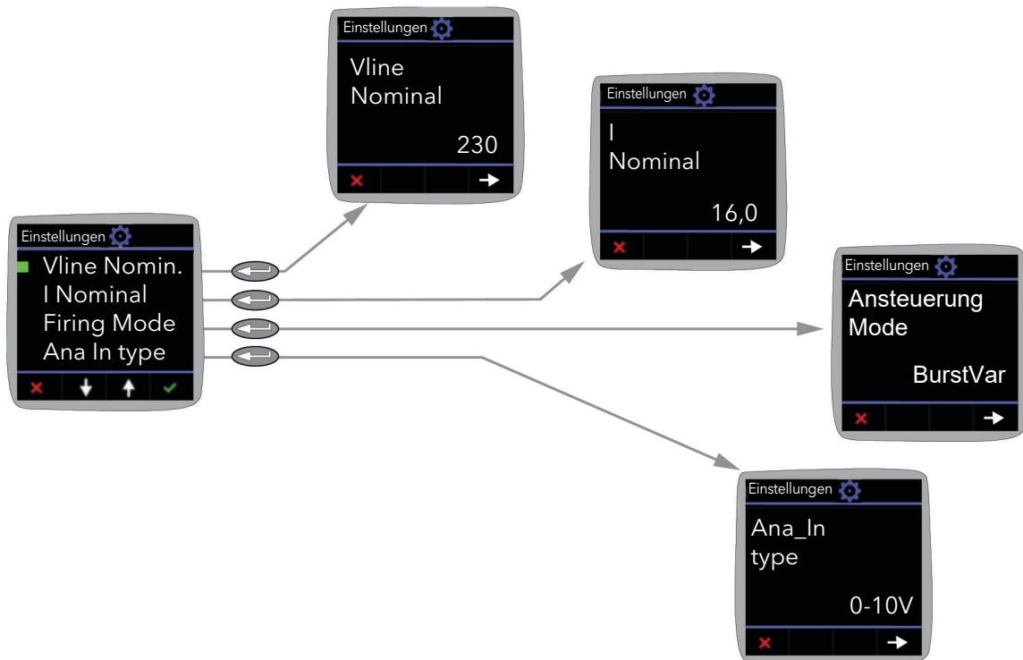
Abbildung 30 Einstellungsmenü
