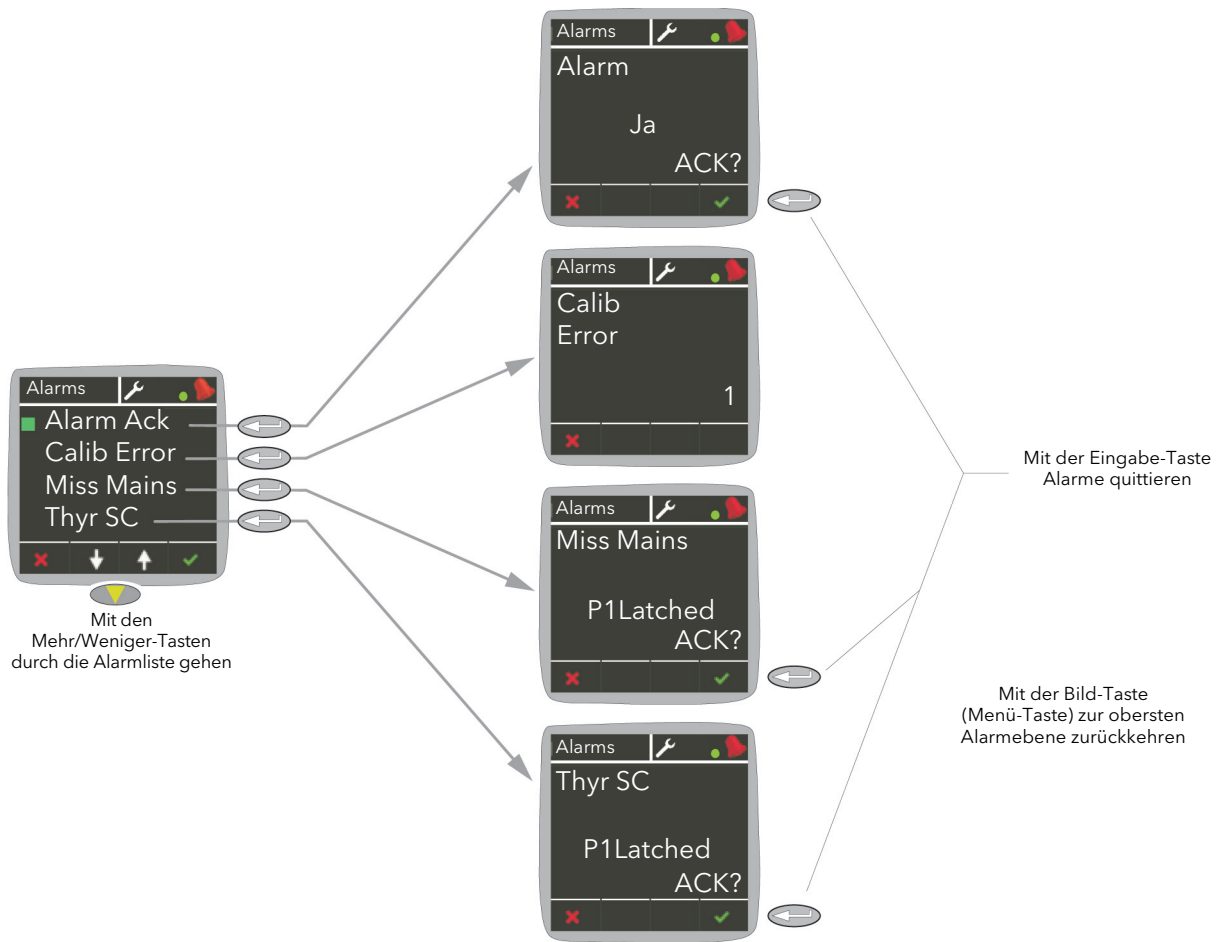
Abbildung 24 Alarmmenü
