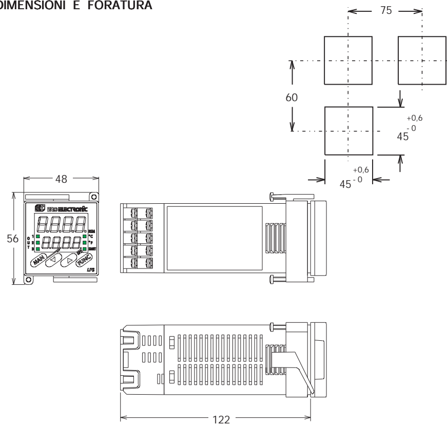
Fig. 2 DIMENSIONI E FORATURA
