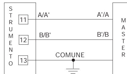
Fig. 12 - COLLEGAMENTO DELL'INTERFACCIA
