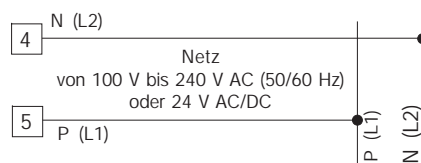
Abb.13 ANSCHLUSS AN DAS STROMNETZ
