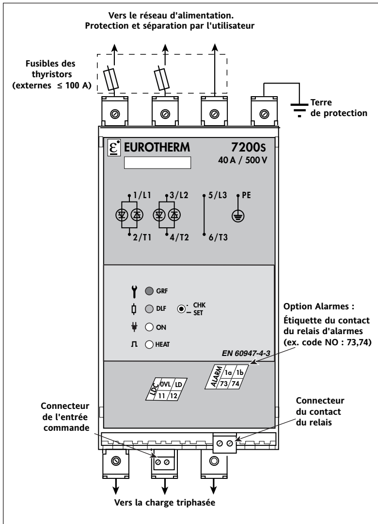
Figure 2-5 Schéma général de branchement pour les unités \leq 100 A
