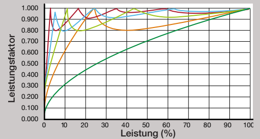
Leistungsfaktor Kurve mit n Anzapfungen.
