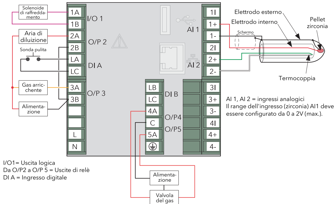
Figura 4.11.3 Tipico collegamento di una sonda zirconia
