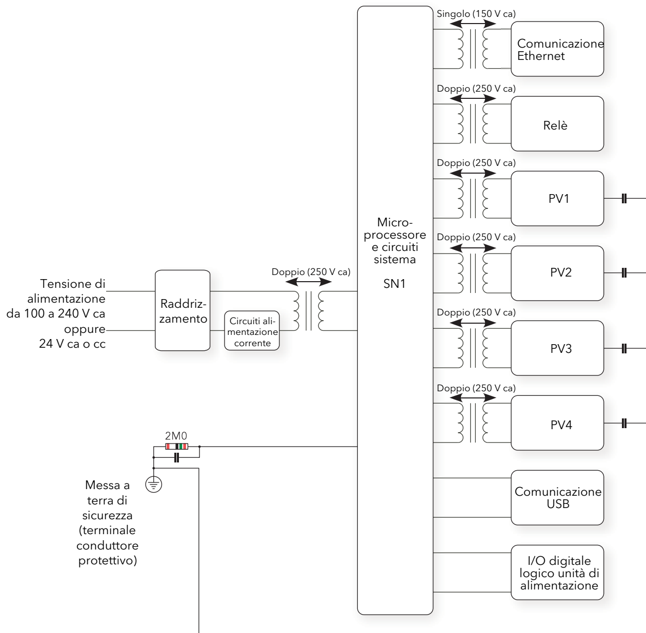
Figura C5 Schema isolamento
