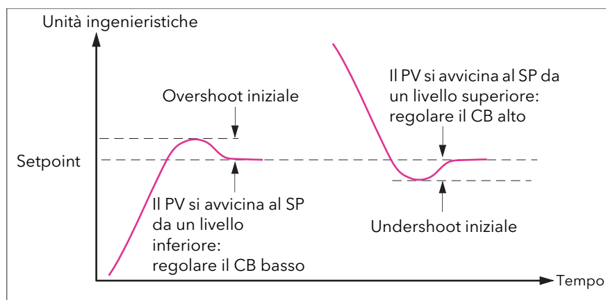
Figura 2.4.6b Impostazione manuale del cutback
