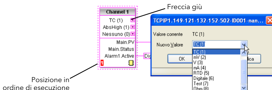
Figura 6.3.2a Esempio di blocco funzione
