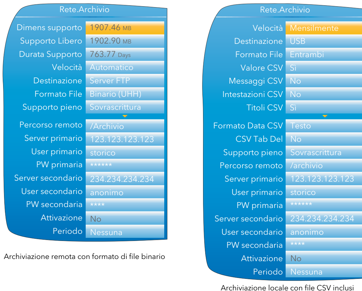
Figura 4.2.2a Configurazione di Archivio non controllata (impostazioni tipiche)
