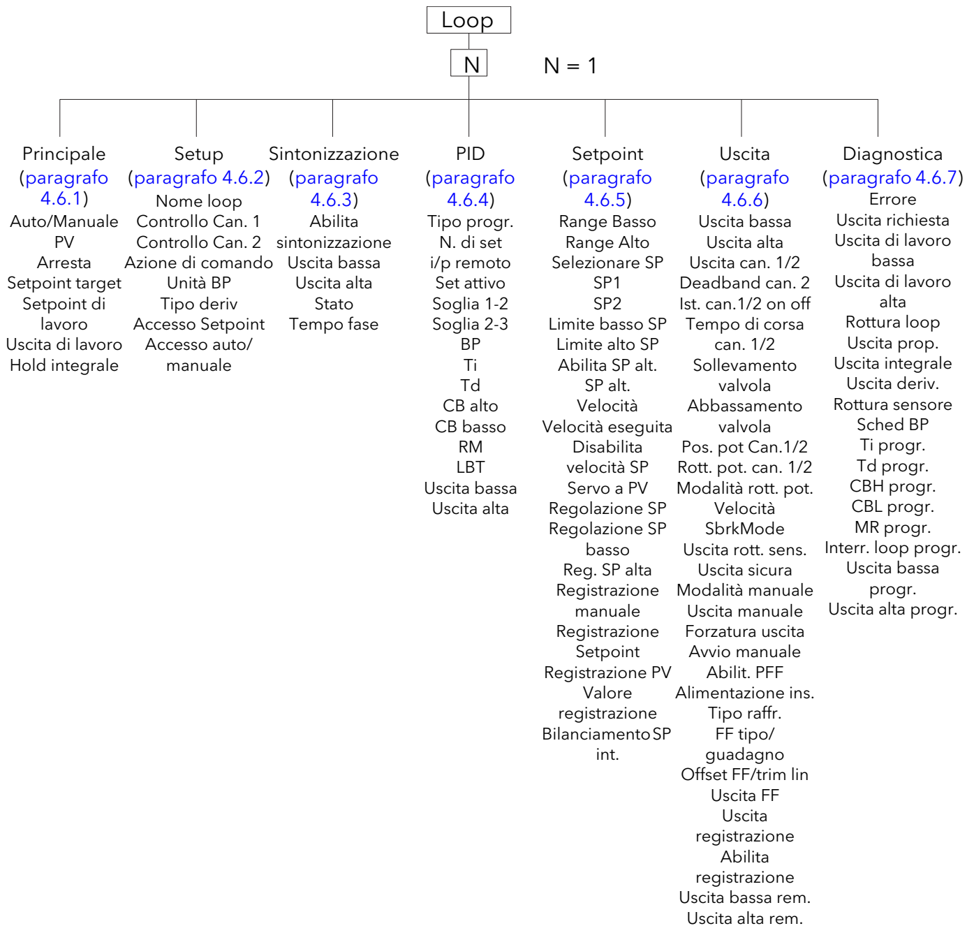
Figura 4.6 Schema di configurazione Loop
