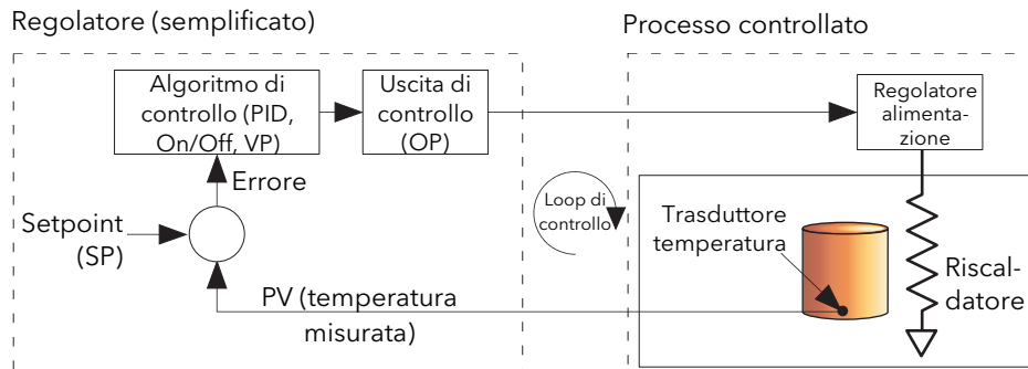
Figura B1.1 Esempio di loop di controllo
