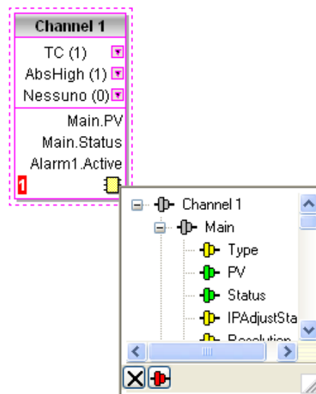
Figura 6.3.2c Finestra di dialogo di selezione dell'uscita
