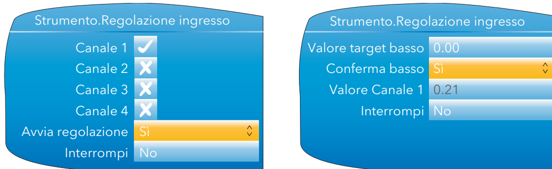
Figura 4.1.8c Procedura di regolazione del canale (2)
