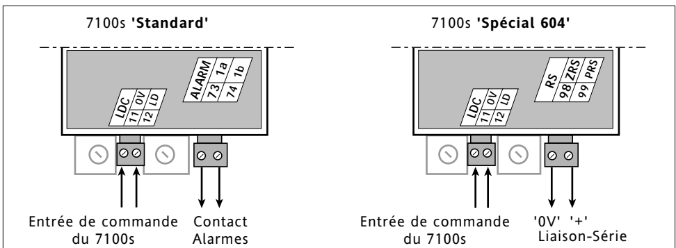
Figure 2-4 Branchement de la Liaison-Contact et Liaison-Série
