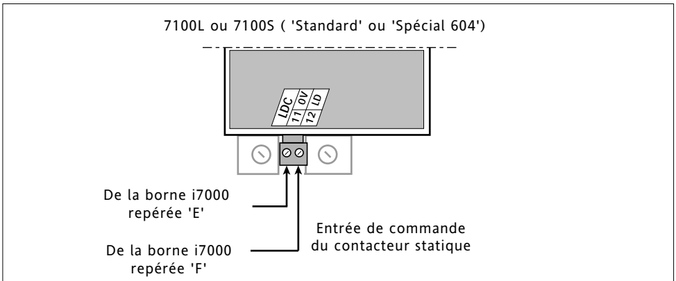
Figure 2-3 Branchement de la Commande Logique des contacteurs statiques 7000
