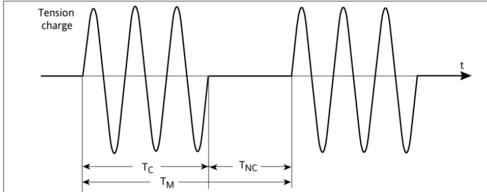
Figure 4-1 Conduction des thyristors en mode «Train d'ondes» (déclenchement au zéro de tension)
