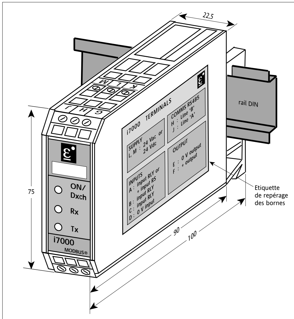
Figure 2-1 Dimensions et Fixation de l'Interface i7000
