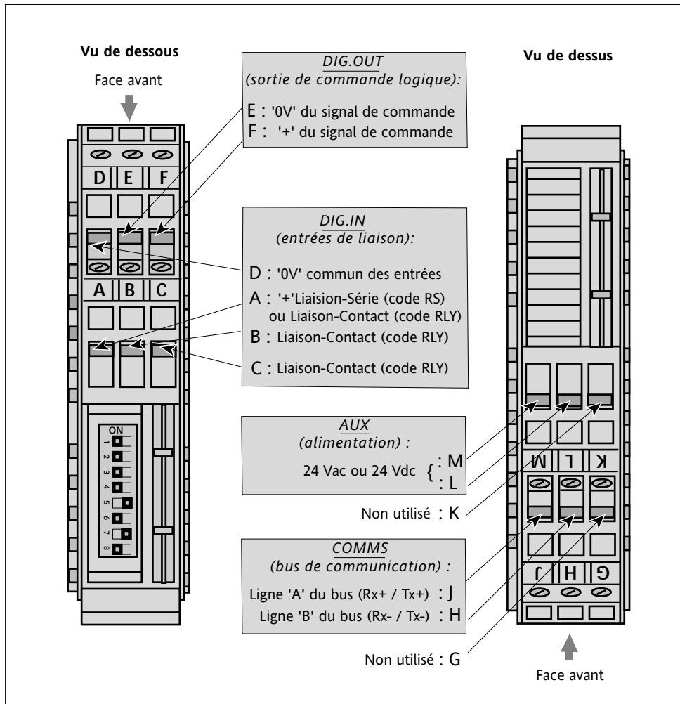
Figure 2-2 Disposition des bornes et des repères de l'Interface i7000 (vus de dessous et de dessus)
