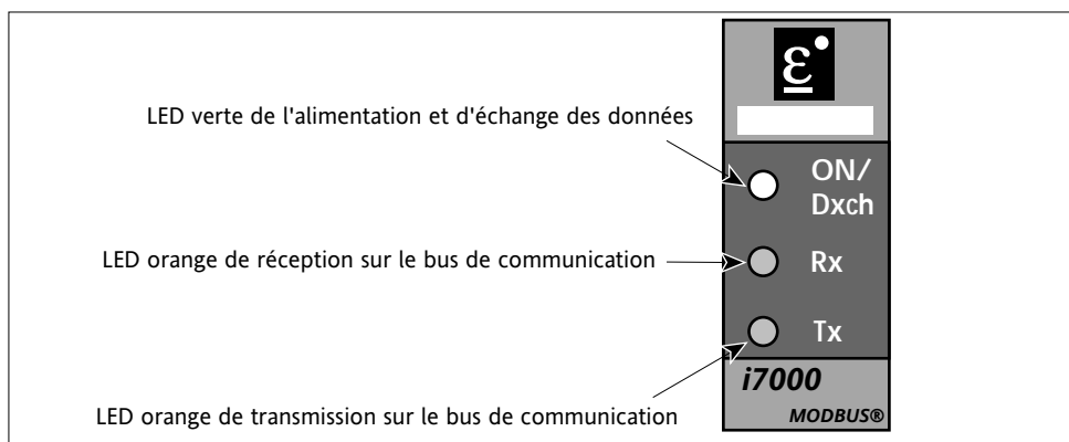
Figure 3-11 LED's de diagnostic de l'état de l'Interface
