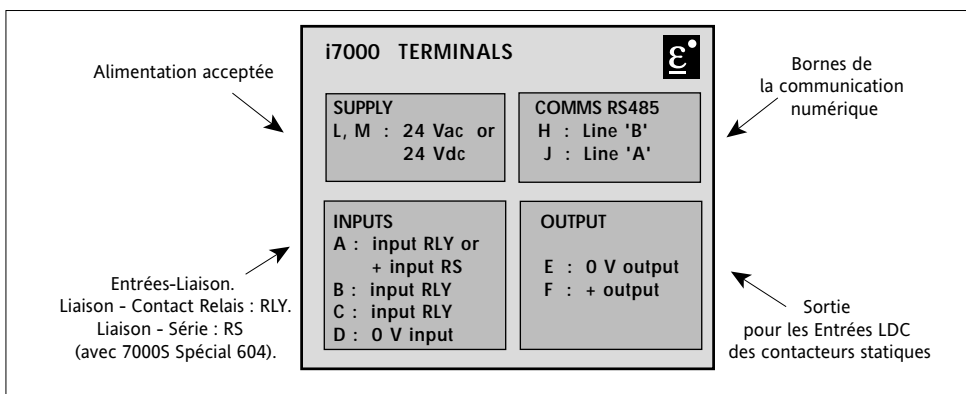
Figure 1-3 Étiquette de repérage des bornes de l'Interface i7000
