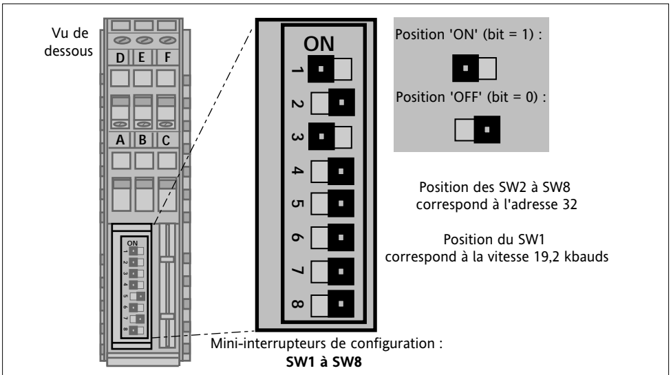
Figure 3-2 Exemple de configuration d'adresse et de la vitesse par les mini-interrupteurs
