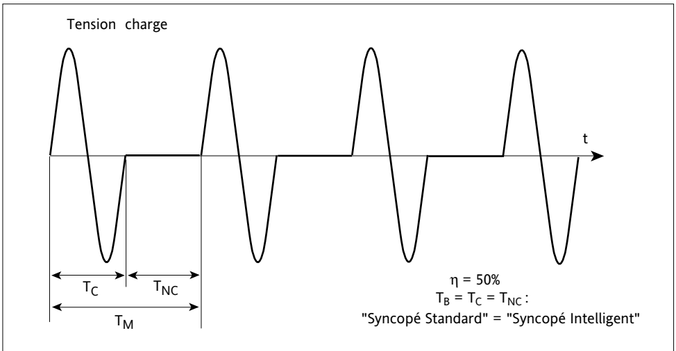
Figure 4-2 Exemple de conduction avec le rapport cyclique \eta = 50\% ( T_B = T_C = T_{NC} ) en modes «Syncoié » et «Syncoié Intelligent»
