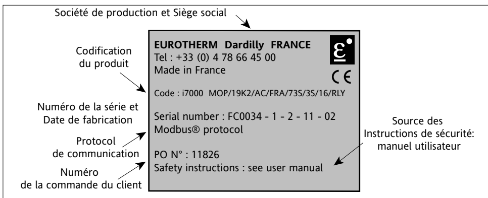
Figure 1-2 Exemple de l'étiquette d'identification (correspond à l'Exemple N°1 de codification)
