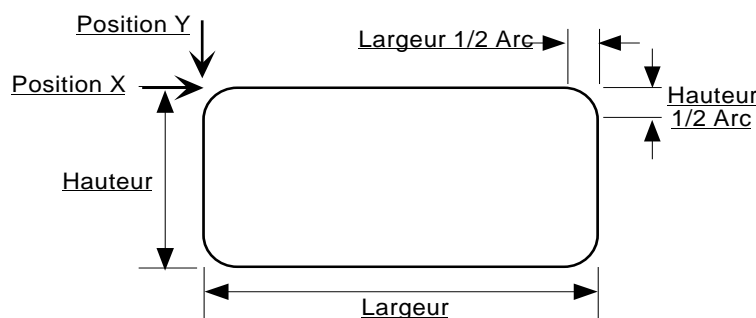
Figure 2.4.14 Définition d'un rectangle arrondi
