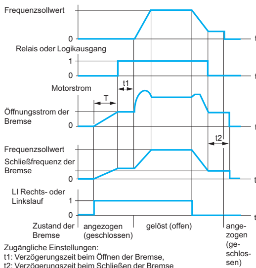
Bremslogik
