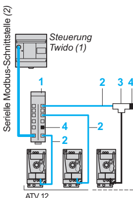
Anschlussschema Modbus, Anschlüsse über Abzweigdosen und RJ45-Steckverbinder
