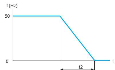
Lineare Auslauframpe
