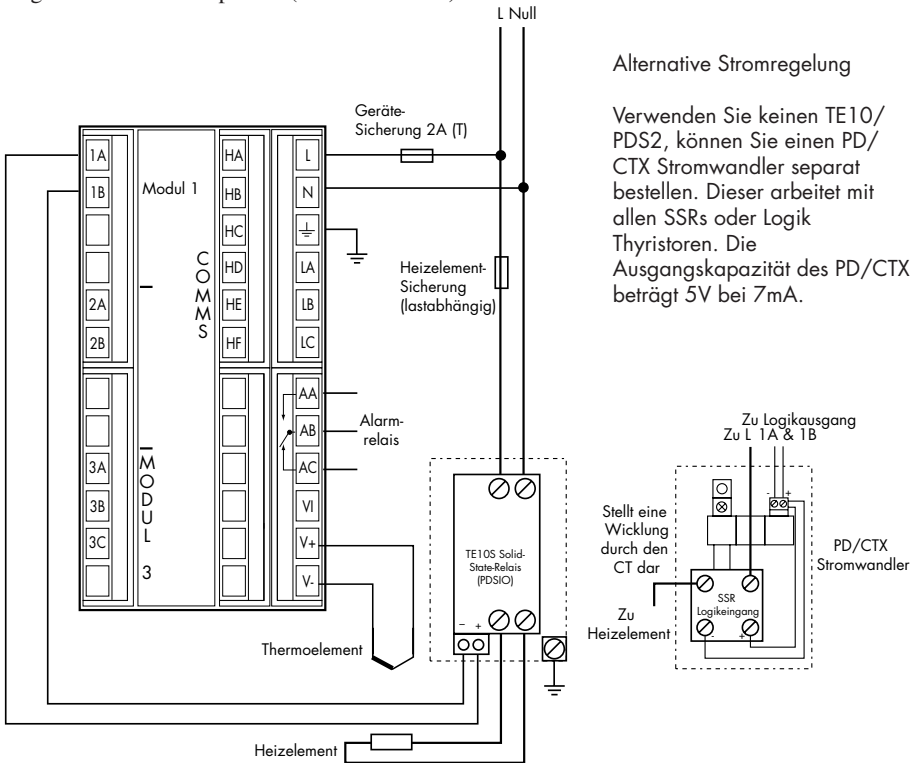
Abbildung D-1 Anschlüsse für Mode 1 und 2
