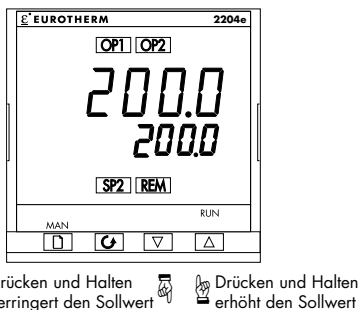
Abbildung 2-4 Einstellen des Sollwertes 2204e
