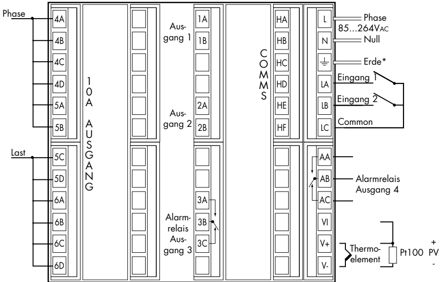
Abbildung 1-6 Rückansicht 2204e
