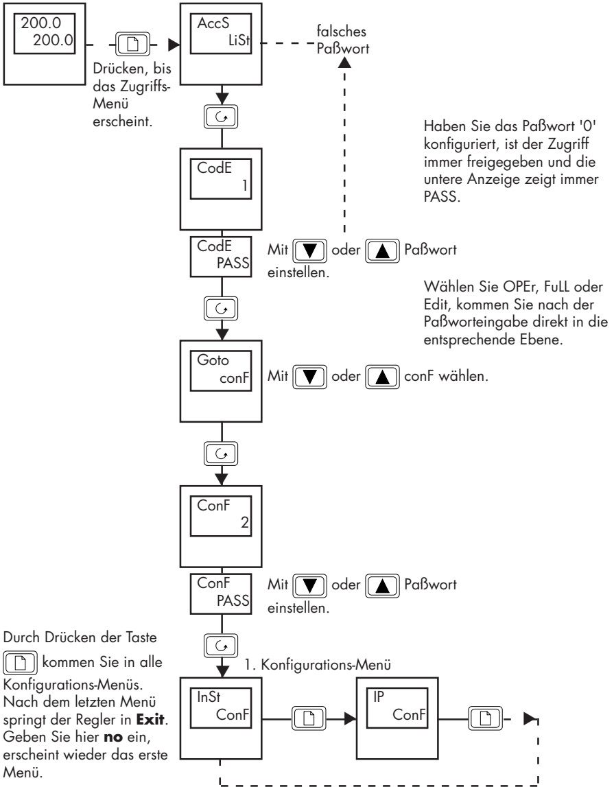
Abbildung 5-1 Auswahl der Konfigurationsebene
