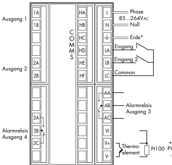
Abbildung 1-5 Rückansicht 2208e
