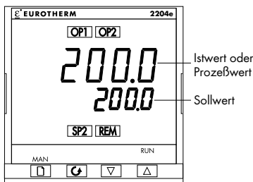
Abbildung 2-3 Hauptanzeige 2204e
