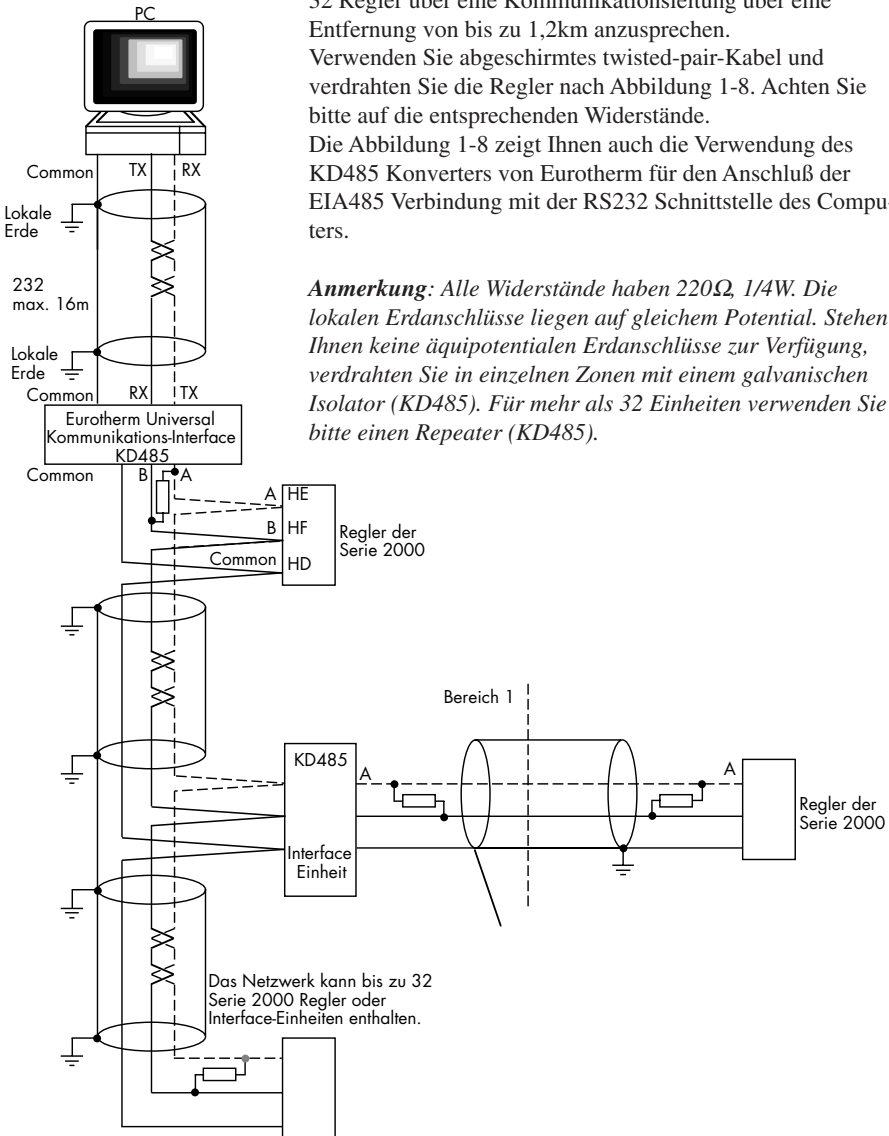
Abbildung 1-8 RS485 Verdrahtung
