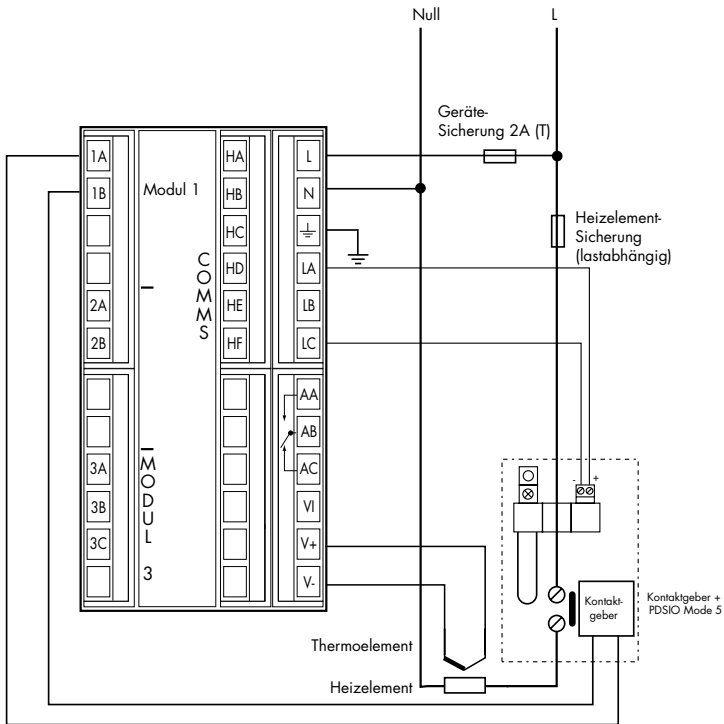
Abbildung D-2 Anschluß für Mode 5
