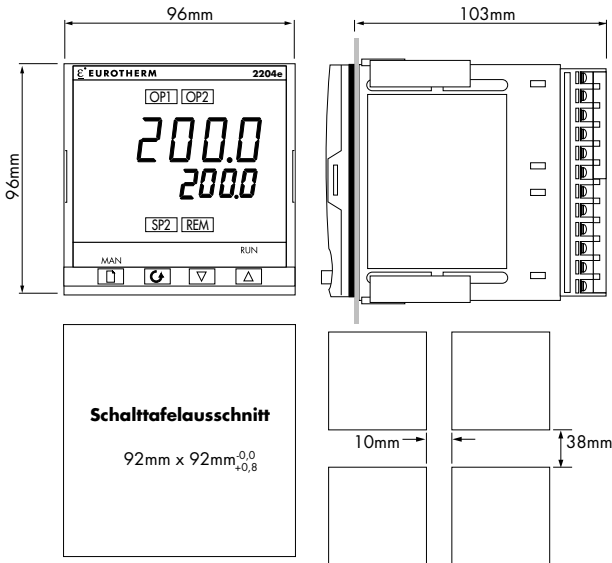
Abbildung 1-4 Abmessungen und Mindestabstände 2204e
