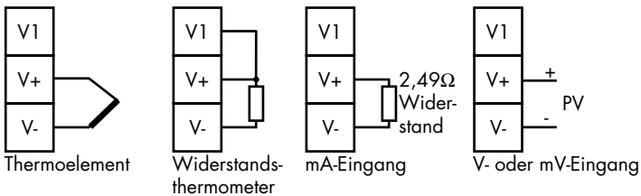
Abbildung 1-7 Sensoreingang
