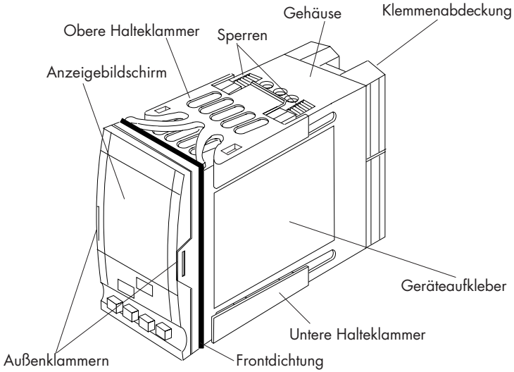
Abbildung 1-1 Reglermodell 2208e
