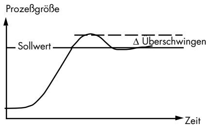
Abbildung 4-2 Cutback Low: Anfahrversuch, Istwert &lt; Sollwert
