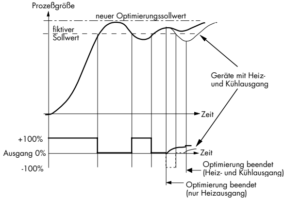
Abbildung 4-1 Selbstoptimierung
