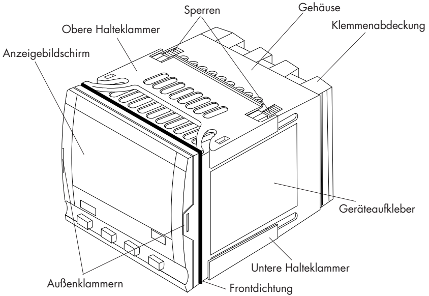
Abbildung 1-2 Reglermodell 2204e
