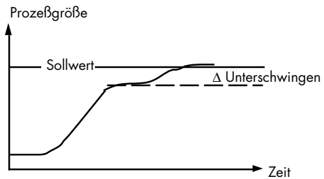
Abbildung 4-2 Cutback Low: Anfahrversuch, Istwert &lt; Sollwert
