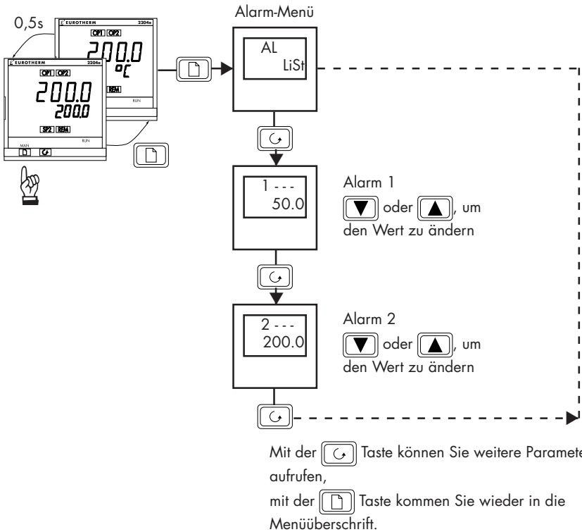
Abbildung 2-8 Parametermenüs
