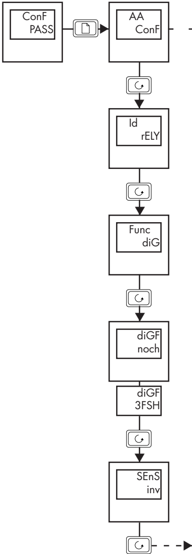
Abbildung 7-2 Zuweisen eines Ausgangs
