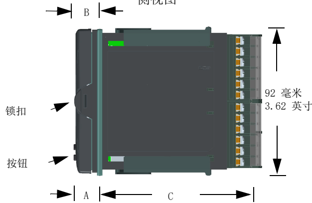
侧视图
