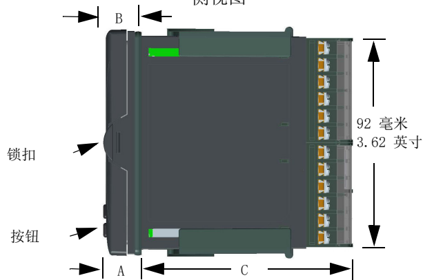
侧视图
