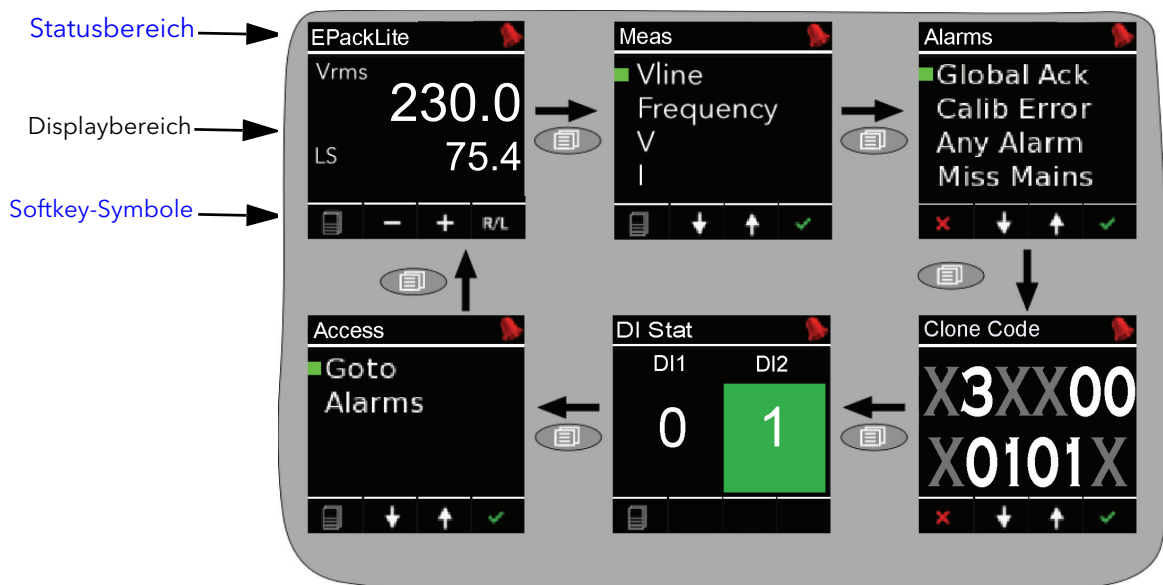
Abbildung 15 Bedienoberfläche
