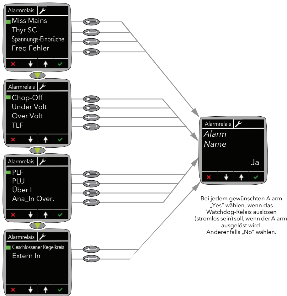
Abbildung 32 Alarmrelaismenü
