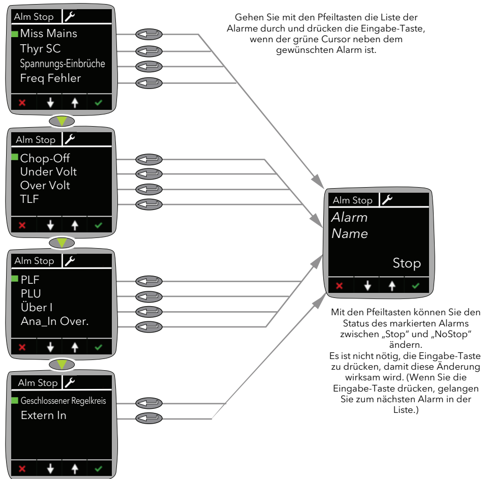
Abbildung 31 Alarmstoppmenü
