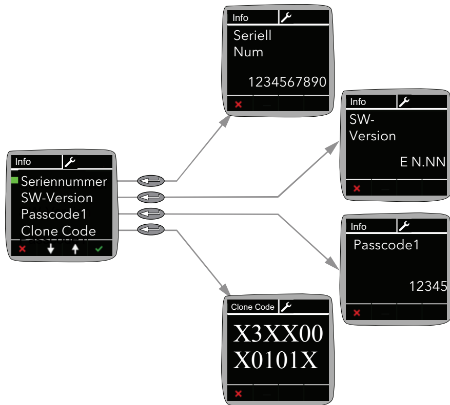
Abbildung 27 Infomenü
