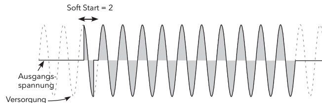
Abbildung 23 Beispiele für Sicherheitsrampen (Impulsgruppenbetrieb)
