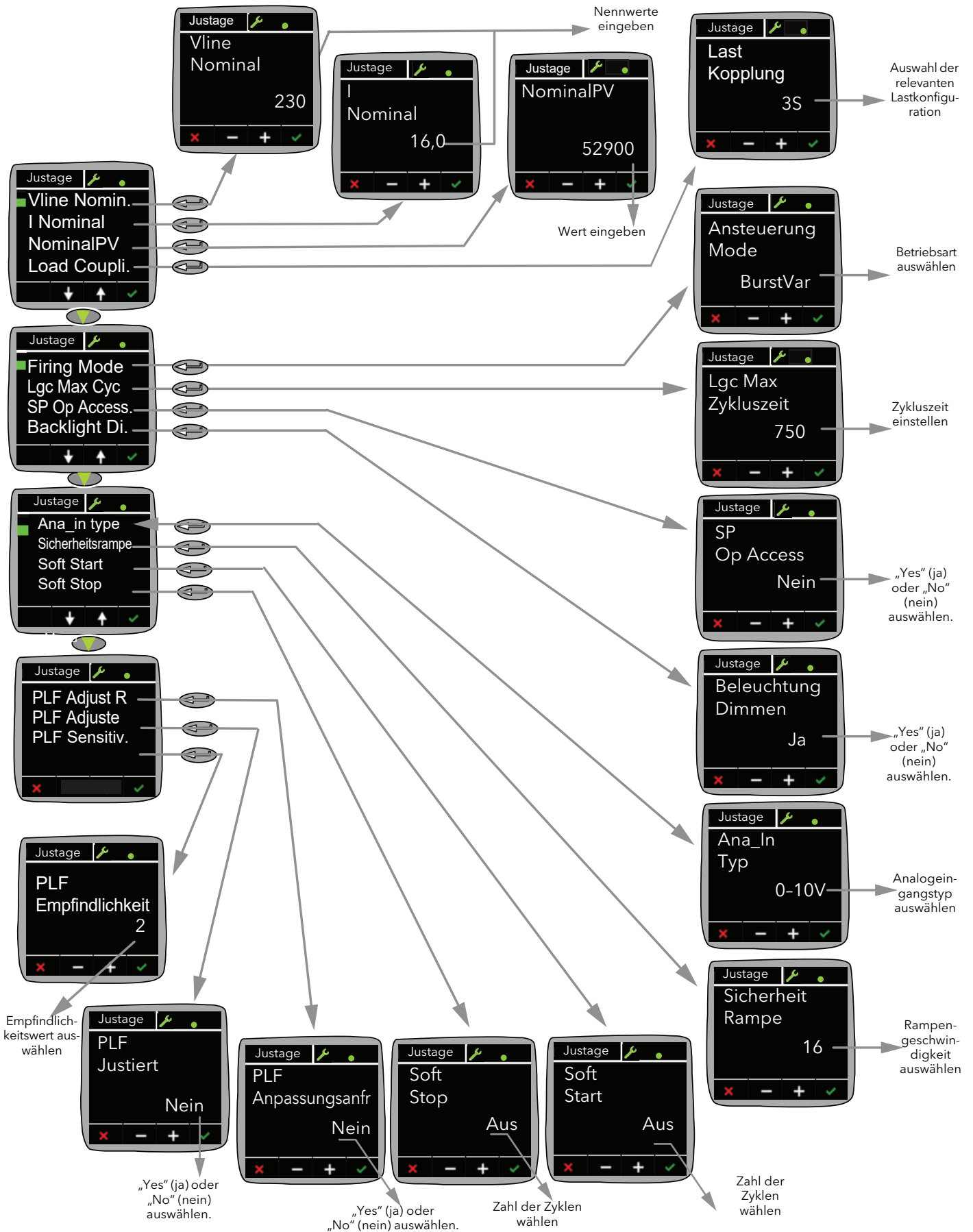
Abbildung 22 Adjust-Menü
