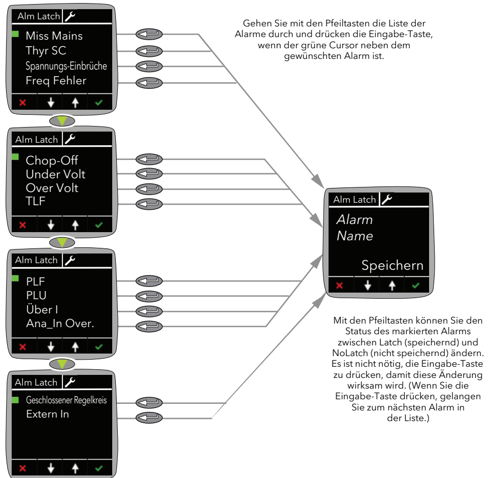
Abbildung 30 Alarmspeichermenü
