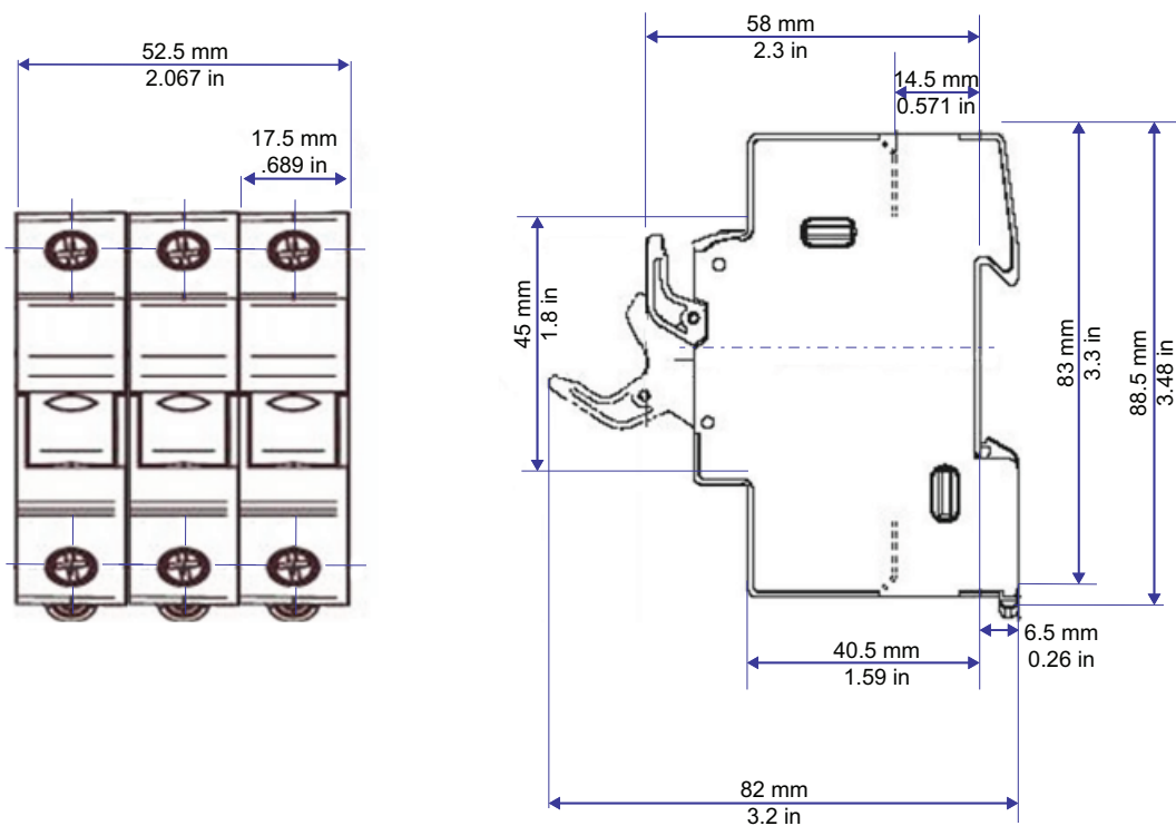
Abbildung 36 Sicherungshalterabmessungen: US103 (10x38 mm)
