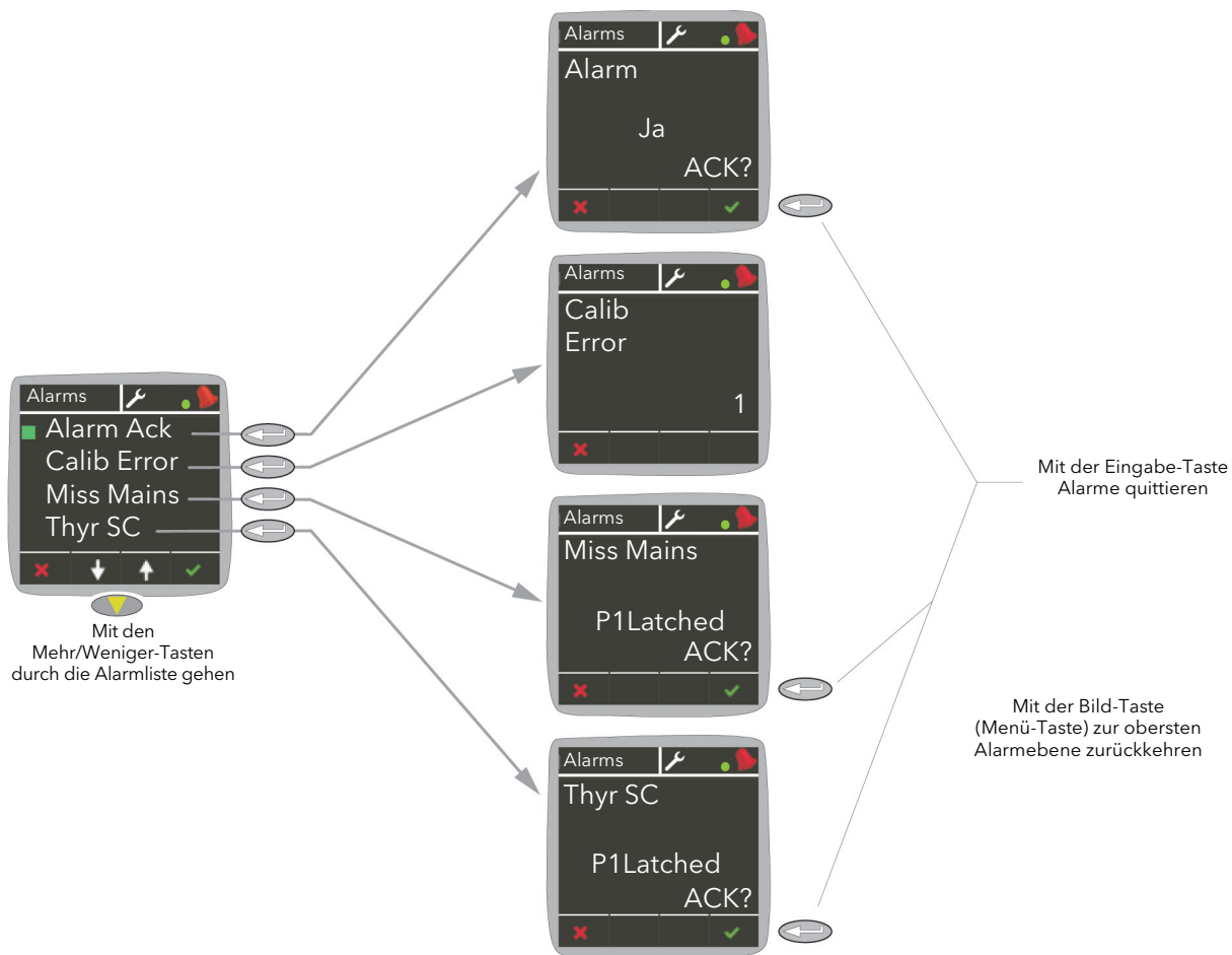
Abbildung 28 Alarmmenü
