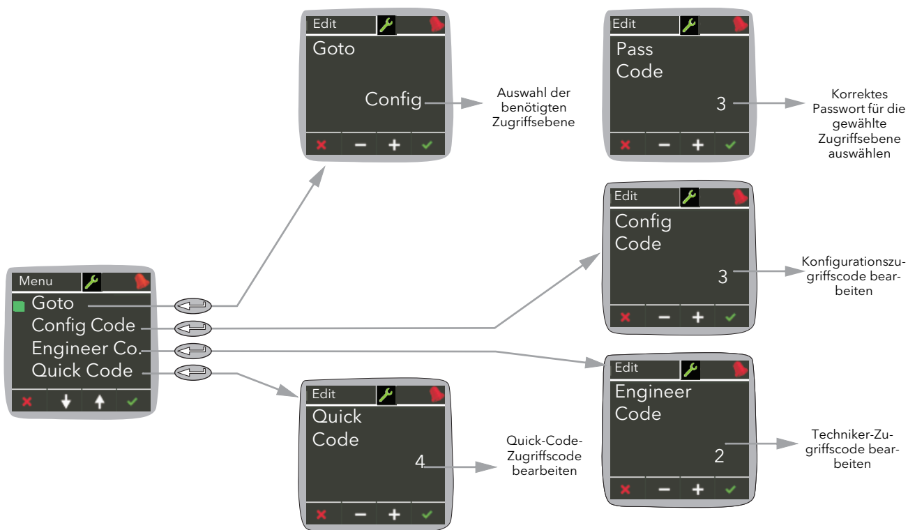
Abbildung 35 Zugriffsmenü
