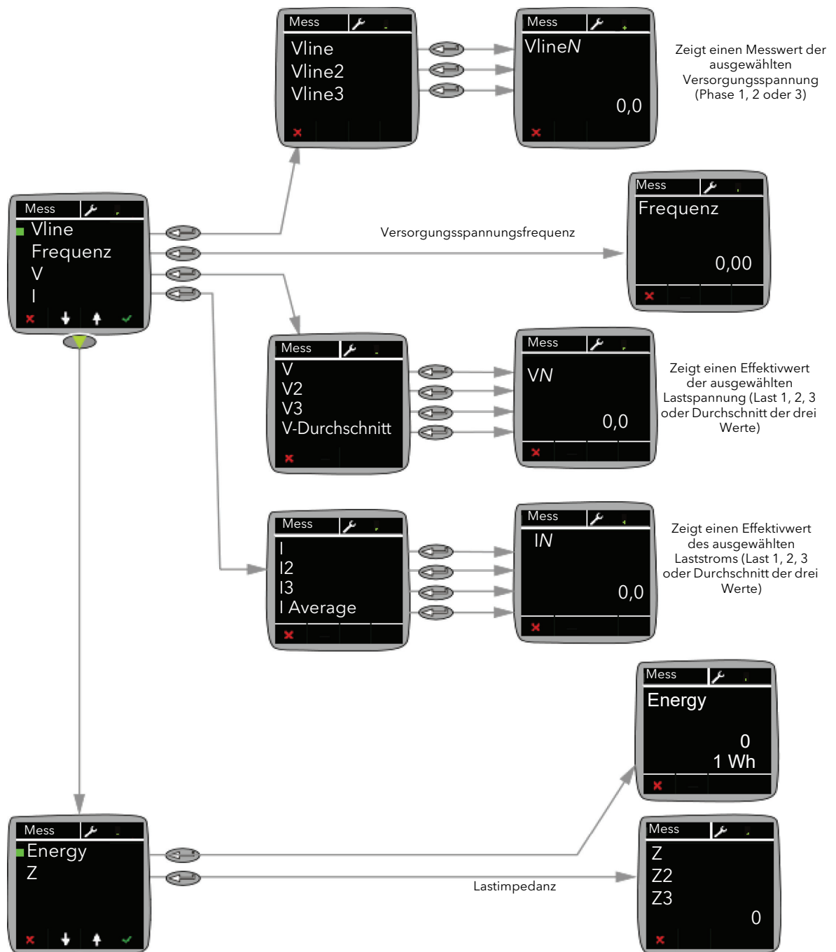
Abbildung 21 Messwert-Menü
