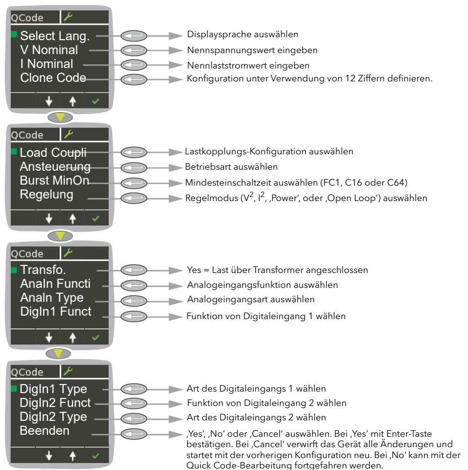
Abbildung 16 Typisches Quick Code-Menü
