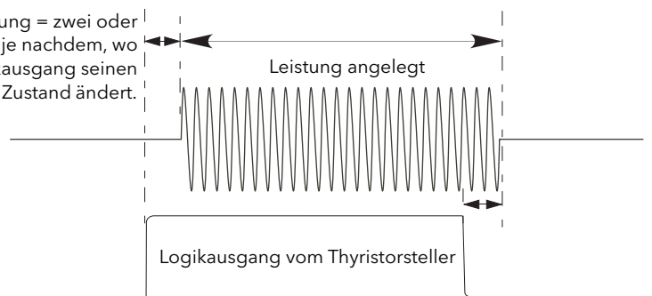
Abbildung 17 Logikbetrieb
