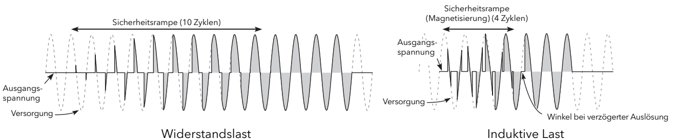
Abbildung 23 Beispiele für Sicherheitsrampen (Impulsgruppenbetrieb)
