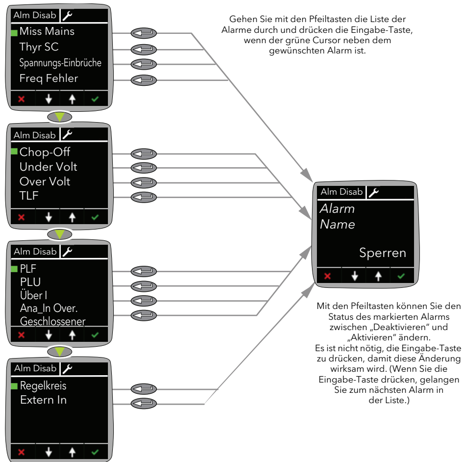
Abbildung 29 Alarmdeaktivierungsmenü
