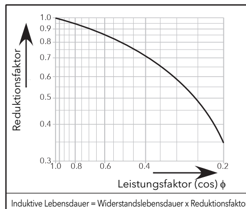
Abbildung 41 Relaisminderungskurven
