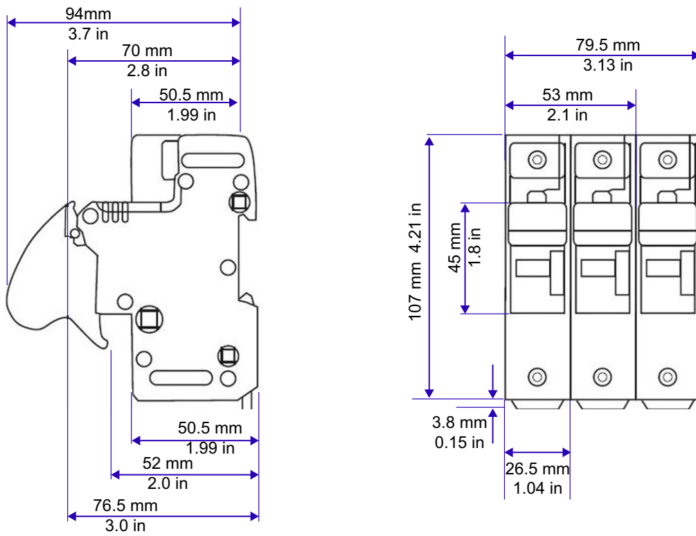
Abbildung 38 Sicherungshalterabmessungen: US143 (14x51 mm)
