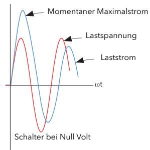
Abbildung 25 Definition bei verzögerter Auslösung
