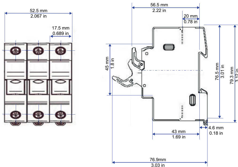
Abbildung 37 Sicherungshalterabmessungen: CUS103 (10x38 mm)
